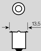
P13,5s IEC 7004-40
