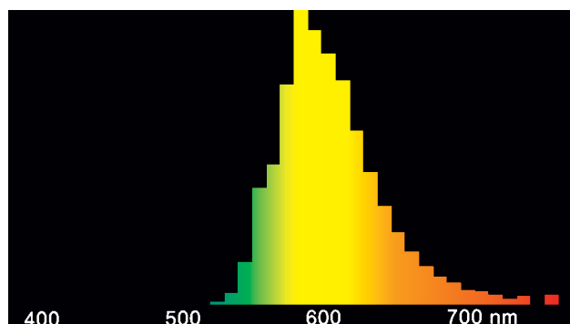
Spektralfördelningskurva ljusfärg 62
