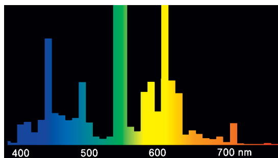
Spektralfördelningskurva Ljusfärg 840 SPS
